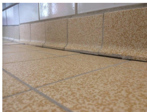
Hohlkehlen-Fliese FALSCH verlegt (stehend). Wasser kann bei undichter Silikon-Fuge in die Mauer eindringen
