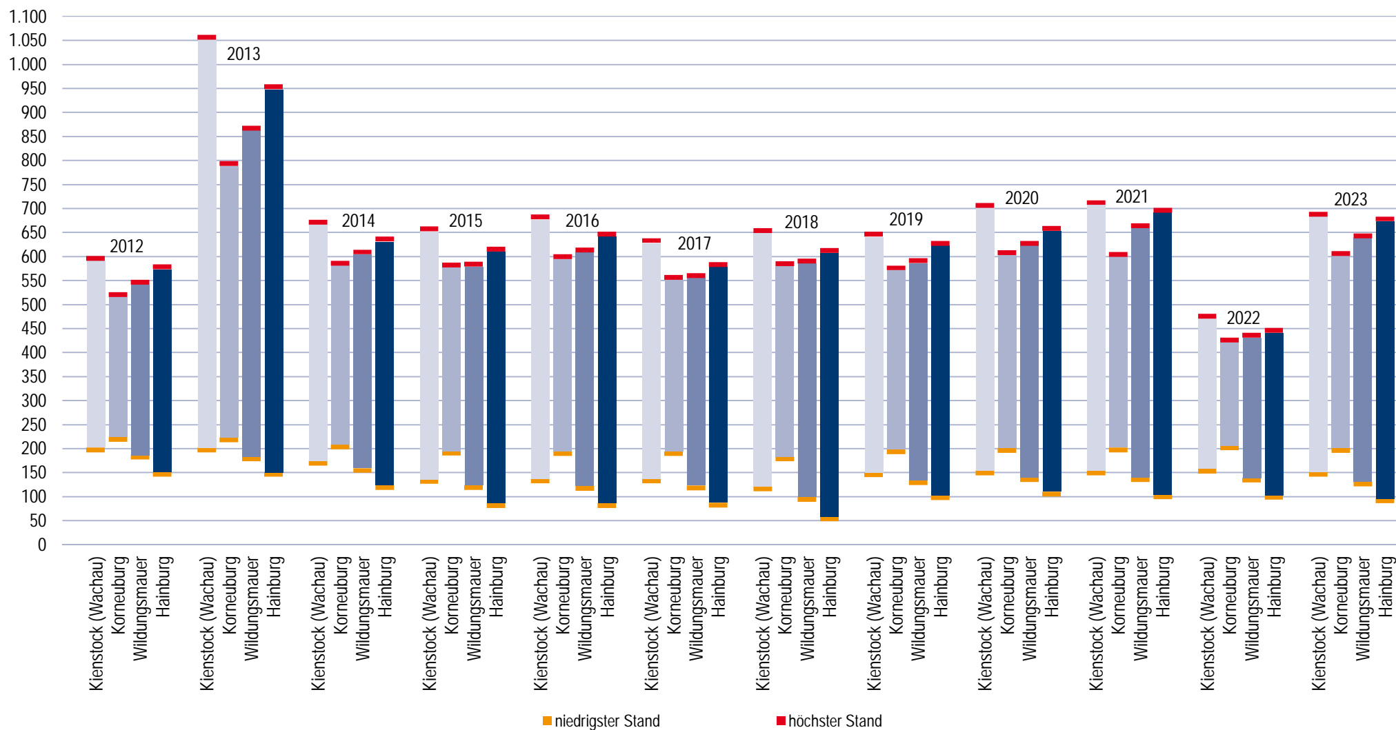
Tagesmittelwerte Wasserstand (in cm)
